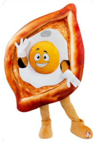
Hačapuri
